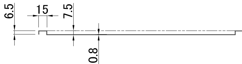
A-A 断面図
