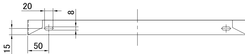
A矢視図
