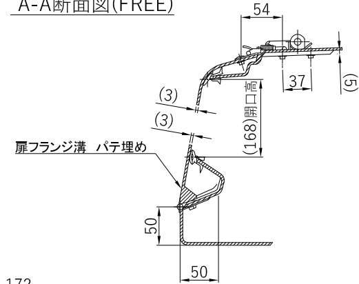
A-A断面図(FREE)
