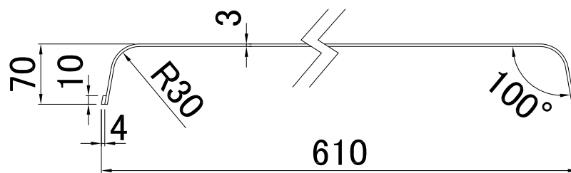
A-A断面图
