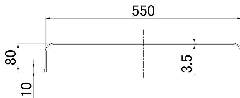
A-A断面图
