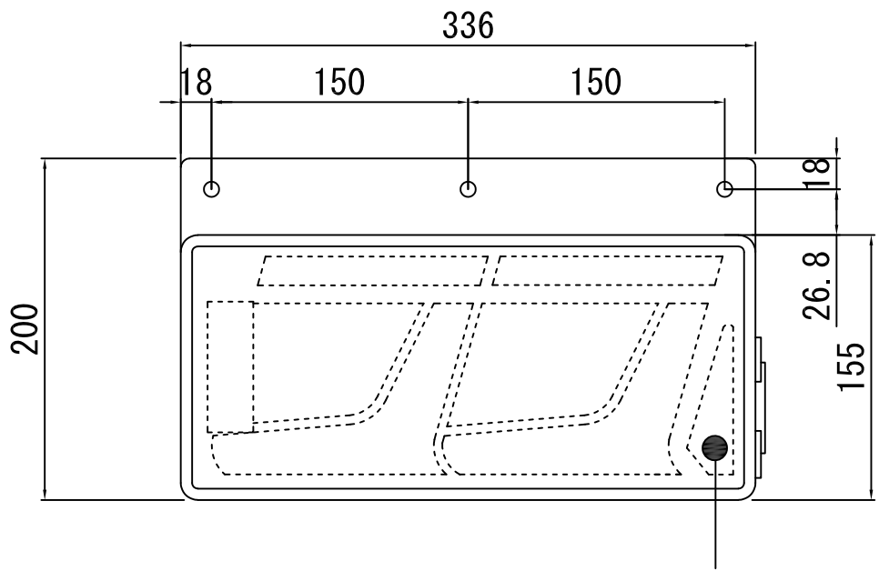
E13 UN (ECE) 認可マーク位置 (インナーレンズ)
