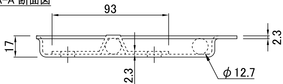
A-A 断面图
