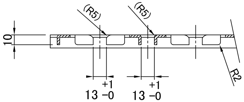
A-A 断面
