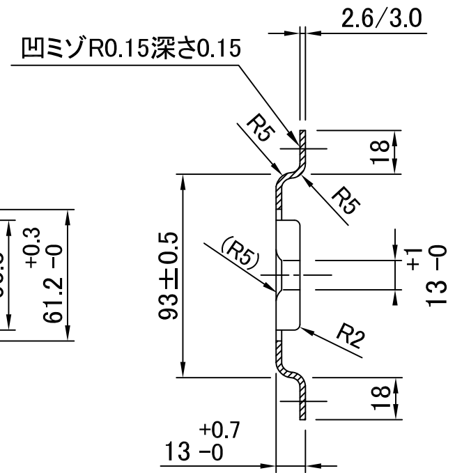
B-B 断面
