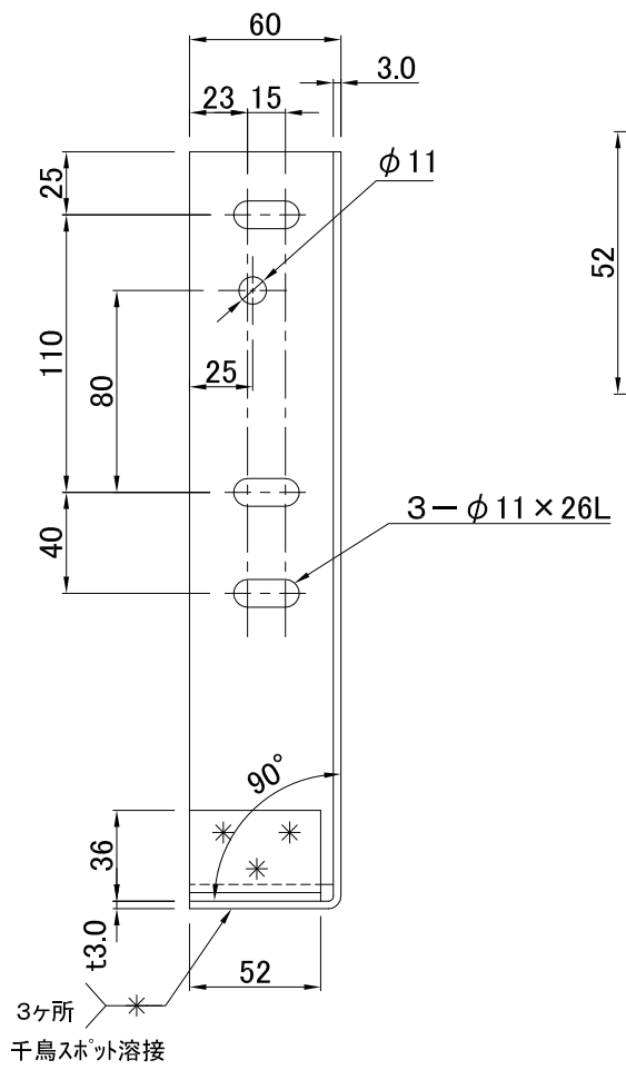
2. 補強詳細図 (拡大図)
