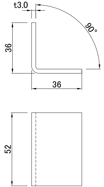
2. 補強詳細図 (拡大図)
