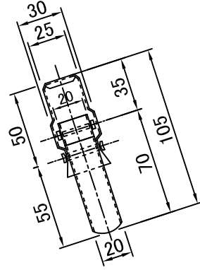
キャッチ部拡大図
