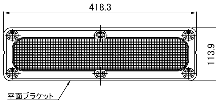
平面ブラケット取付図
