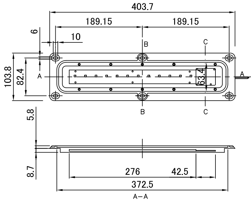
平面ブラケット取付図
