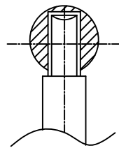
A-A 断面図 (S=1:1)
